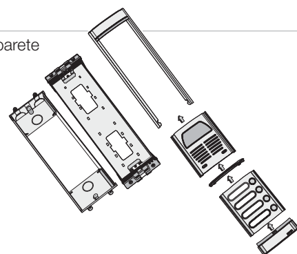
Incasso parete con cornice parapioggia
